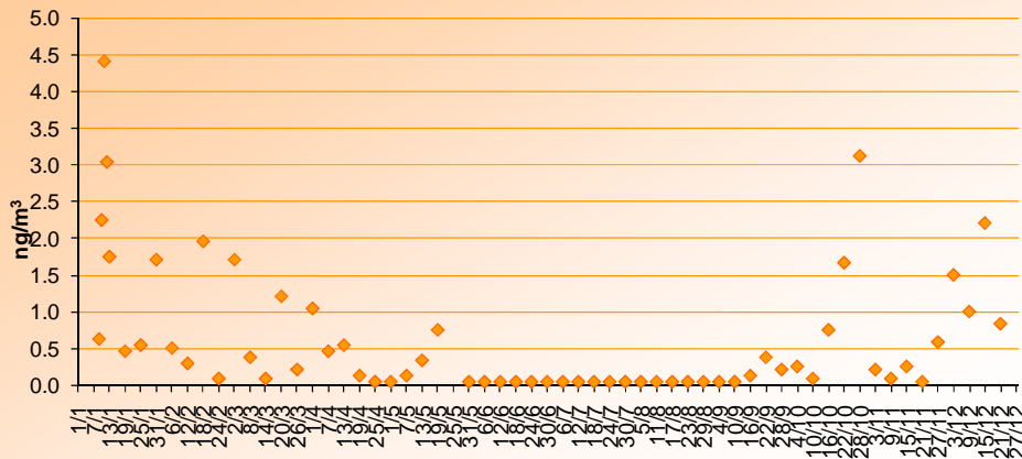
Concentration journalière du benzo(a)pyrène mesuré au niveau du site "Mairie" à Bourbonne-les-Bains (52) en 2010
