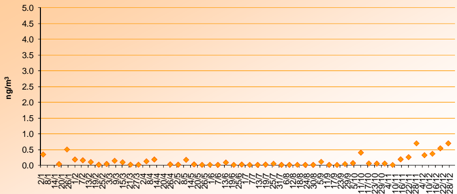
Concentration journalière du benzo(a)pyrène mesuré au niveau de la station MERA à Revin (08) en 2010
