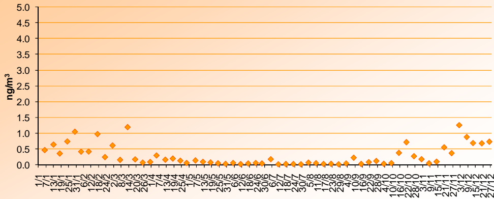
Concentration journalière du benzo(a)pyrène mesuré au niveau du site "Ecole" à Montcy-Notre-Dame (08) en 2010
